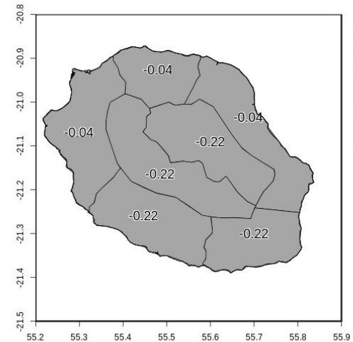
Score RPSS: RR_7ZONES DJF-2020 It1
