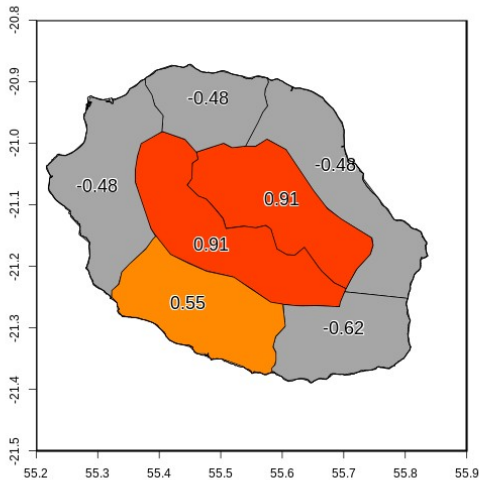
Score RPSS: RR_7ZONES OND-2020 It1
