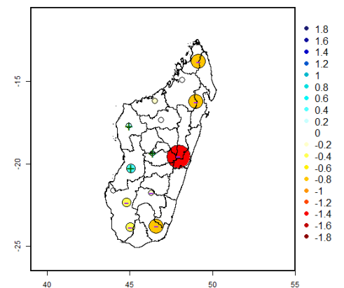
RR Std. Anom.: DJF 2020
