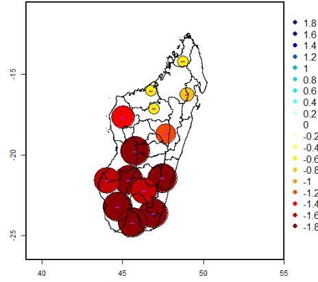
RR Std. Anom.: NDJ 2020
