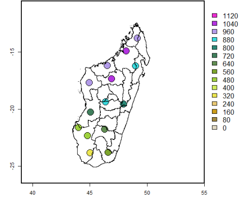
RR Avg.: DJF
