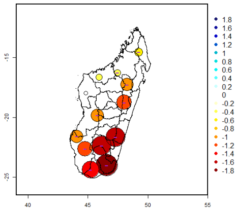
RR Std. Anom.: OND 2020
