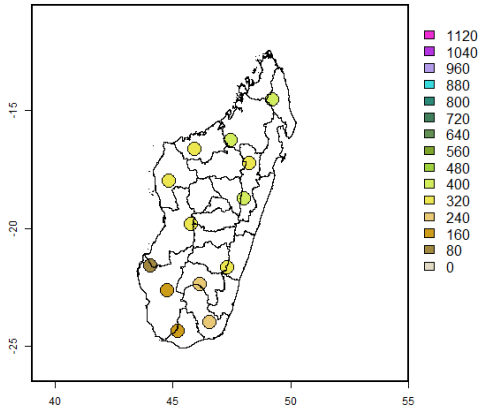
RR Avg.: OND
